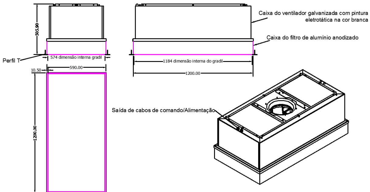
Figura 3: Esboço do Equipamento
