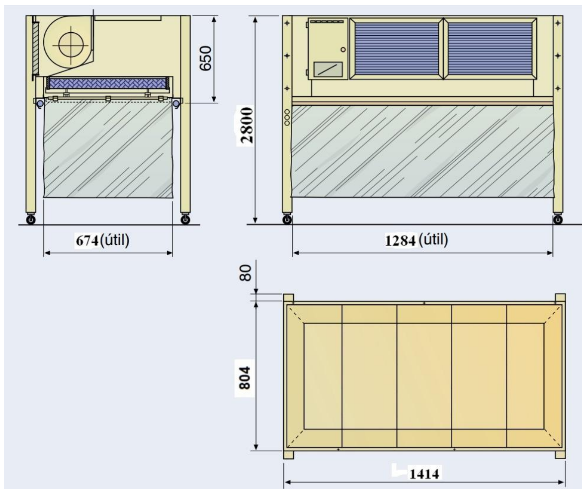
Figura 2: Esboço do Equipamento
